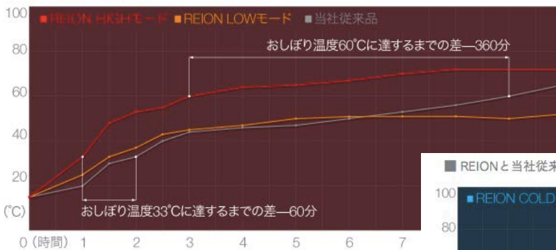
■ REIONと当社従来品との加温性能比較 ※1 ※2 ※3
