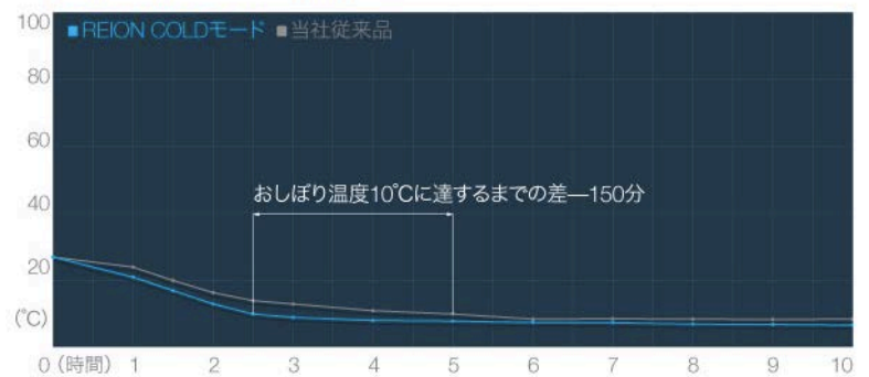
■ REIONと当社従来品との冷却性能比較 ※1 ※4
